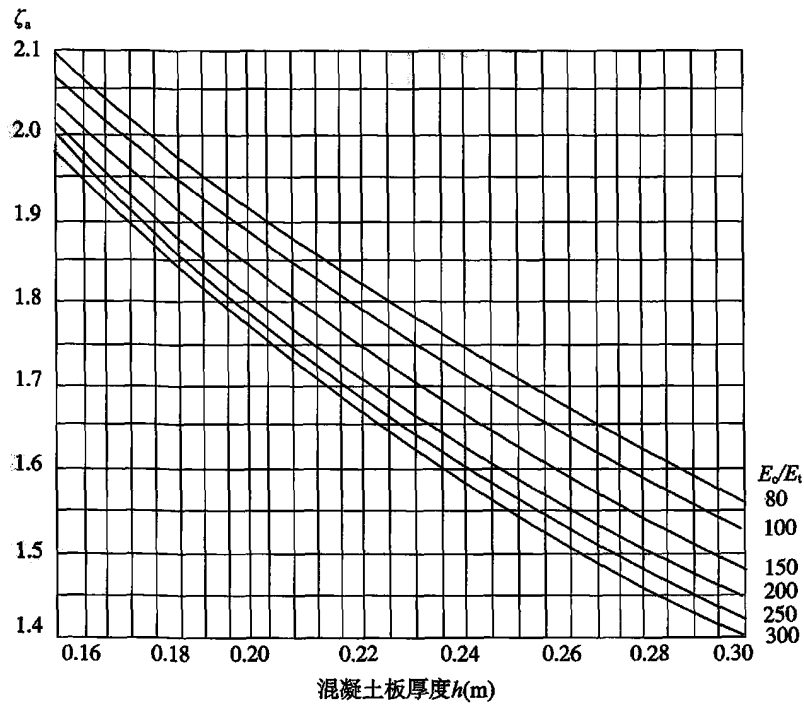
图 C.1.2 系数 \zeta_a 图
