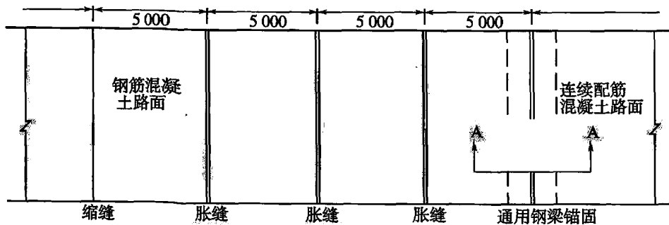
图 5.5.4-1 钢筋混凝土地梁锚固 (尺寸单位: mm)
