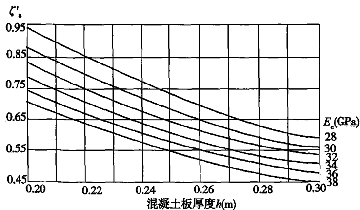
图 C.2.1 系数 \zeta'_a 图
